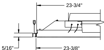
Frame NR (Narrow Regress)
