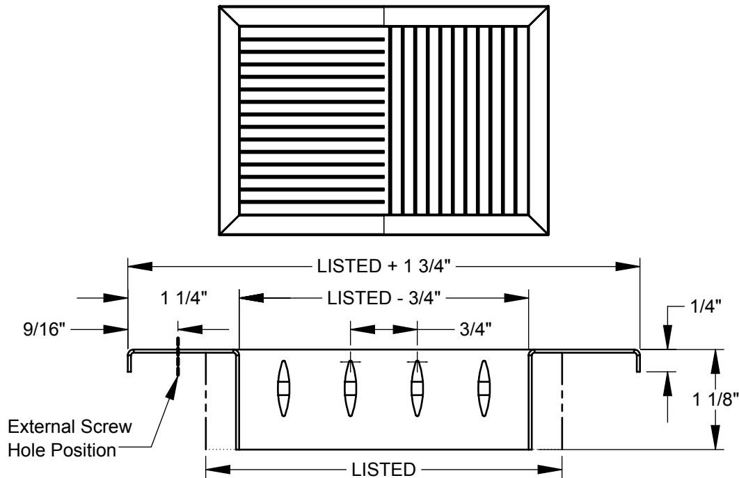
AVS50 - Horizontal Blades
