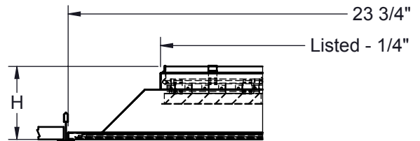
Margin LT, Lay-in T-Bar
